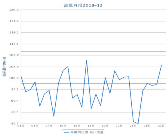
12月月流量曲线
